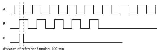
Incremental encoder
